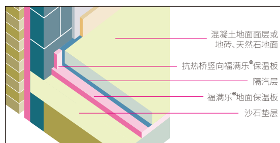
建筑地面保温构造简图
