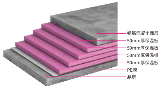
地面构造剖面图
