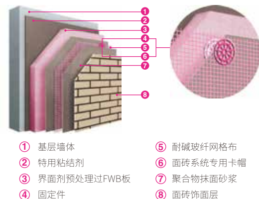
系统结构
