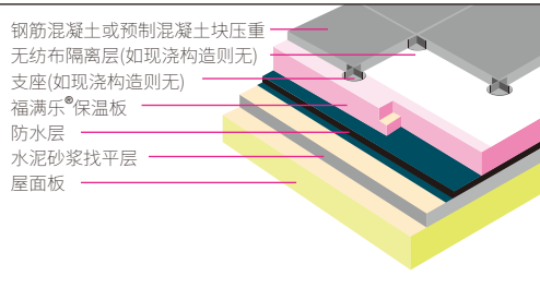
钢筋混凝土或预制混凝土块压重构造简图
