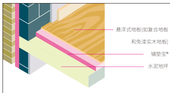
铺垫宝®保温构造简图
