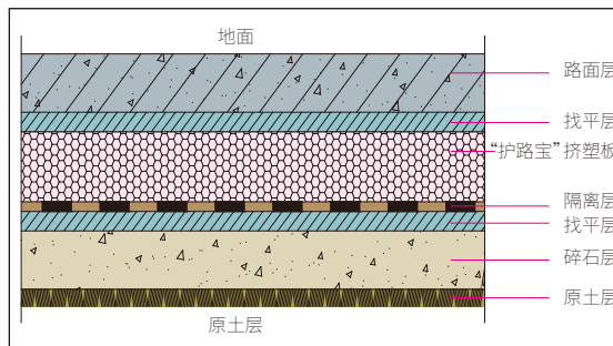
冻土地面常规作法
