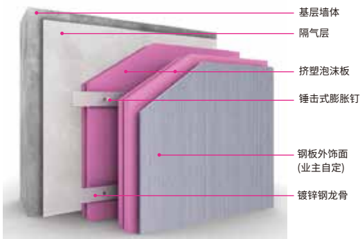
墙面构造剖面图
